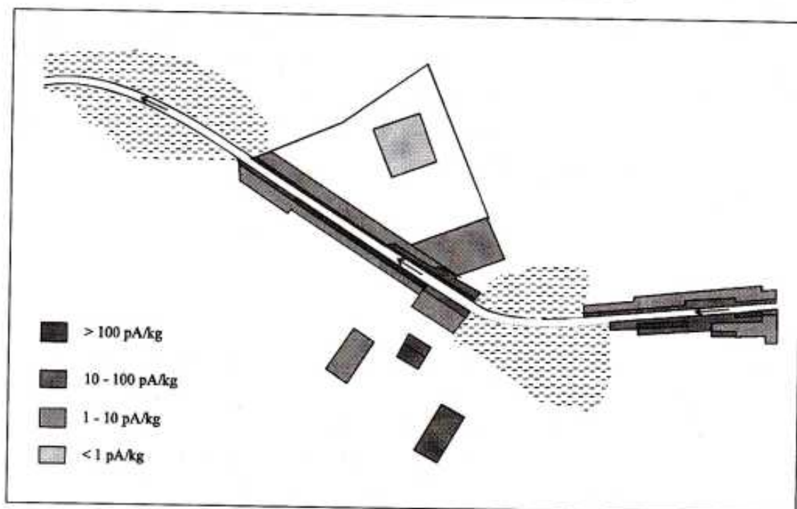
Ryc. 2. Moc dawek promieniowania gamma w pobliżu cieku Gamma radiation in the vicinity of river channel
