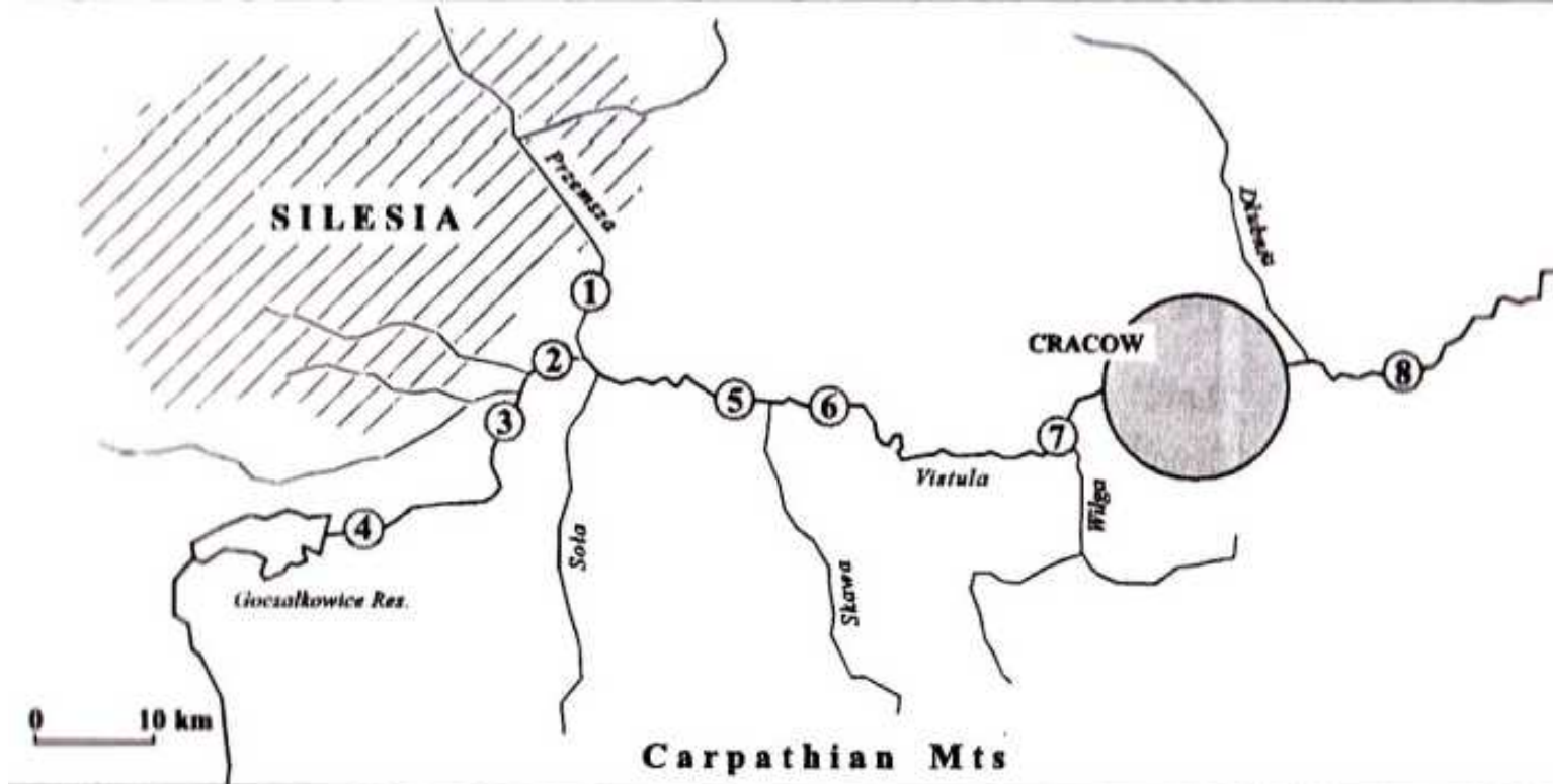
Ryc. 1. Lokalizacja punktów poboru osadów rzecznych Location of river sediment sampling sites
